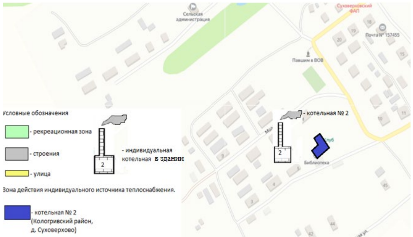
Рисунок 3. Схема индивидуального источника теплоснабжения в д. Суховерхово
